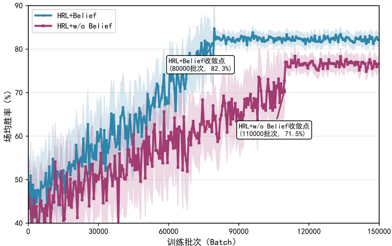
信念估计模块对收敛速度的影响对比（对战RuleRobot+RuleRobot）
